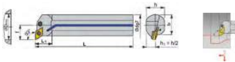
Abb.: Rechtsausführung Lieferung ohne Wendeschneidplatten.
