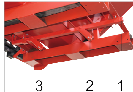
3 automatische Entriegelungspunkte.
