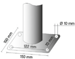
4 Dübelbefestigung
