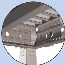
Hauptträger
