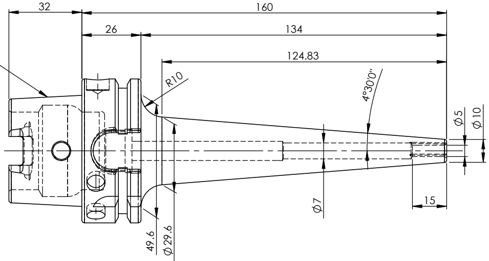
SECTION A-A SCALE 3 : 1
